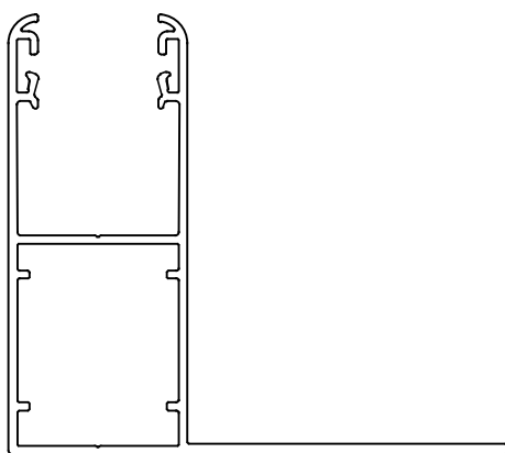
CR 53x22 L60 11624
