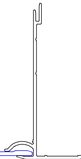
PROFIL ISOLATION EXTERIEURE 12307
